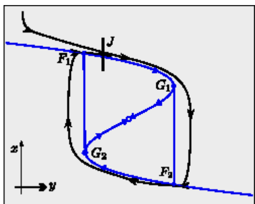
Релаксационный цикл в быстро-медленной системе типа осциллятора Ван дер Поля - по виду это РЕШЕНИЕ сходно с ЛЕТАЮЩЕЙ УТКОЙ
