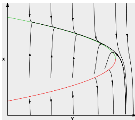
Фазовый портрет быстро-медленной системы зеленым показана устойчивая часть медленной поверхности, красным — неустойчивая - напоминает стаю летящих уток
