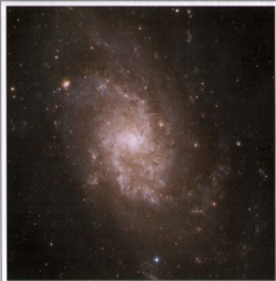
Спиральная галактика M33 в созвездии Треугольник.
