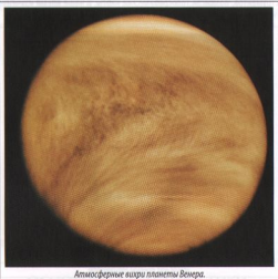
Атмосферные вихри планеты Венера.
