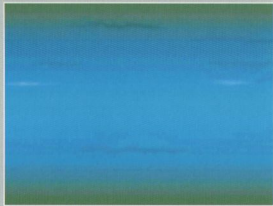
Изображение поверхности Урана, полученное с борта космического зонда «Вояджер-2».
