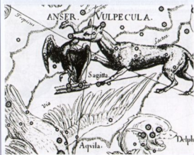
Изображение созвездия Стрелы в атласе «Уранография» 1690 года Яна Гевелия.
