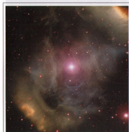
Две планетарные туманности NGC 6164 и NGC 6165 в созвездии Наугольник. Снимок получен с помощью космического телескопа Хаббл.
