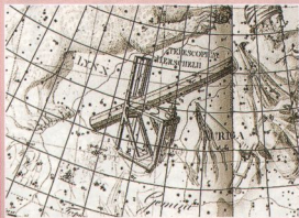
Изображение созвездия Телескоп в атласе «Уранография» 1801 года Иоганна Боде.
