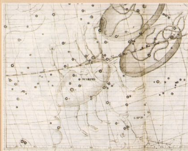
Изображение созвездия Скорпиона в атласе 1729 года Джона Флемстида.
