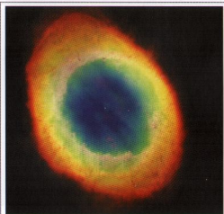
Знаменитая планетарная туманность М57 «Кольцо» из созвездия Лиры.
