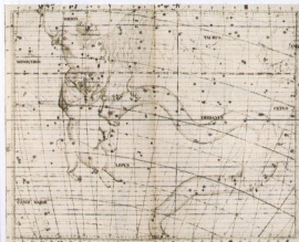
Изображение созвездия Ориона в атласе 1729 года Дюна Флемстида.
