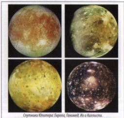
Спутники Юпитера: Европа, Ганимед, Ио и Каллисто.
