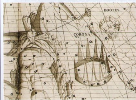
Изображение созвездия Северной Короны в атласе 1729 года Джона Флемстида.
