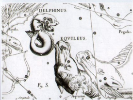
Изображение созвездия Малого Коня в атласе «Уранография» 1690 года Яна Гевелия.
