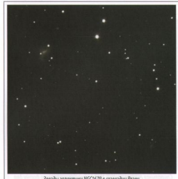
Звезды галактики NGC1679 в созвездии Рысь
