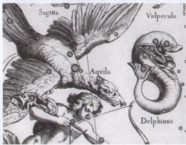
Изображение созвездия Дельфина в атласе 1690 года Яна Гевелия.
