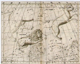
Изображение созвездия Малого Льва в атласе 1729 года Джона Флемстеда.
