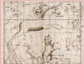
Изображение созвездия Единорога в атласе 1729 года Джона Флемстеда.
