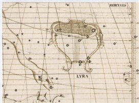
Изображение созвездия Лиры в атласе 1729 года Джона Флемстида.
