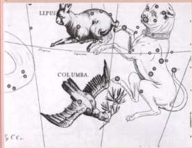
Изображение созвездия Голубя в атласе «Уранография» 1690 года Яна Гевелия.
