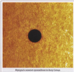
Меркурий в момент прохождения по диску Солнца.
