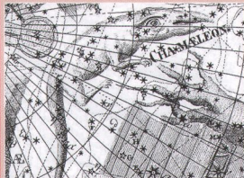
Изображение созвездия Хамелеон в атласе «Уранография» 1801 года Иоганна Баде.
