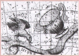
Изображение созвездия Чашы в атласе «Уранография» 1801 года Иоганна Бодя.
