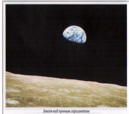
Земля над лунным горизонтом
