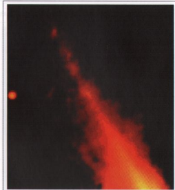
Край пылевого диска вокруг звезды в Живописце. Снимок сделан с помощью телескопа Хаббл.
