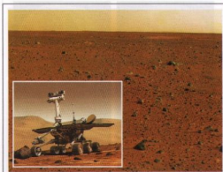
Первая цветная панорама поверхности Марса, переданная на Землю американским марсоходом «Спирит» (внизу).
