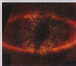
Пылевая диск Фомальгаута. Обрезанные края изображения обусловлены особенностью фотокамеры космического телескопа Хаббл.
