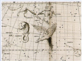
Изображение созвездия Орла в атласе 1729 года Джона Флемстида.
