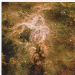
Эмиссионная туманность «Гаргантуй» в созвездии Столовая Гора.
