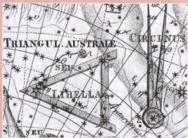
Изображение созвездия Циркуль в атласе «Уранография» 1801 года Иоганна Бодера.
