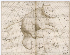
Изображение созвездия Большой Медведицы в атласе 1729 года Джона Флемстида.
