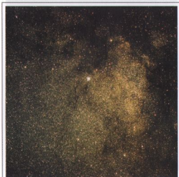
Рассеянное скопление M11 «Дикая Утка» в созвездии Шита.
