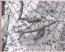
Изображение созвездия Летучей Рыбы в атласе «Уранография» 1801 года Иоганна Байера.
