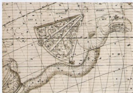
Изображение созвездия Секстант в атласе 1729 года Джона Флемстеда.
