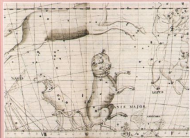
Изображение созвездия Большого Пса в атласе 1729 года Джона Флемстеда.
