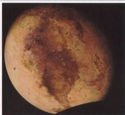
Изображение Плутона, полученное путем реконструкции сведений о планете, известных в настоящее время.
