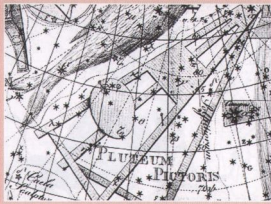
Изображение созвездия Живописца в атласе «Уранография» 1801 года Иоганна Боде.
