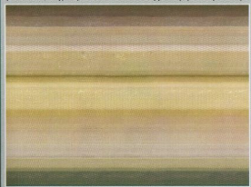
Изображение поверхности Сатурна, полученное с борта космического зонда «Вояджер-2».
