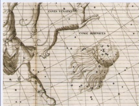
Изображение созвездия Волосы Вероники в атласе 1729 года Джона Флемстада.
