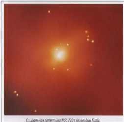
Спиральная галактика NGC 720 в созвездии Кита.
