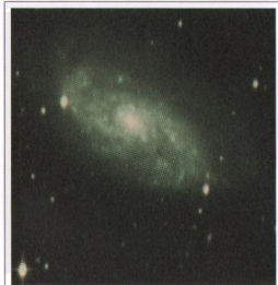
Спиральная галактика NGC 311 в созвездии Чаша.
