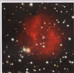
Планетарная туманность Abell 24 в созвездии Малого Пса имеет блеск менее 10 m и видна только в телескоп.
