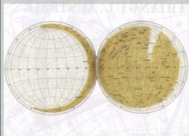
Карта Меркурия. В настоящее время исследована около половины поверхности планеты.
