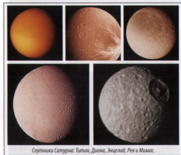
Спутники Сатурна: Титан, Диона, Энцелад, Рея и Мимас.
