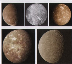
Спутники Урана: Ариэль, Миранда, Оберон, Титания и Умбриэль.
