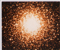
Туманность М30 созвездия Козерог.
