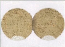
Карта поверхности Венеры.
