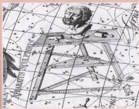
Изображение созвездия Скульптора в атласе «Уранография» 1801 года Иоганна Баде.
