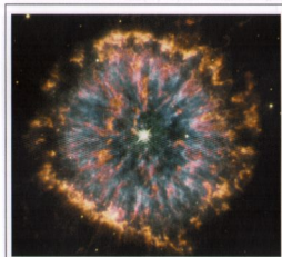
Планетарная туманность NGC 6751 в созвездии Орла напоминает зрачок глаза. Снимок получен с помощью телескопа Хаббл.
