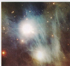
Отражательная туманность Молекулярное облако Хамелеон 1 в созвездии Хамелеон.
