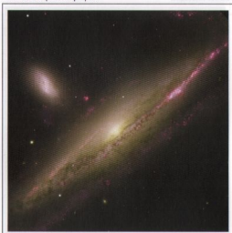
Спиральная галактика NGC 1532 в созвездии Эридана.
