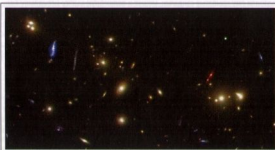
«Дуга Рыси» видна на правой половине снимка в виде наклонной дуги красного цвета.
