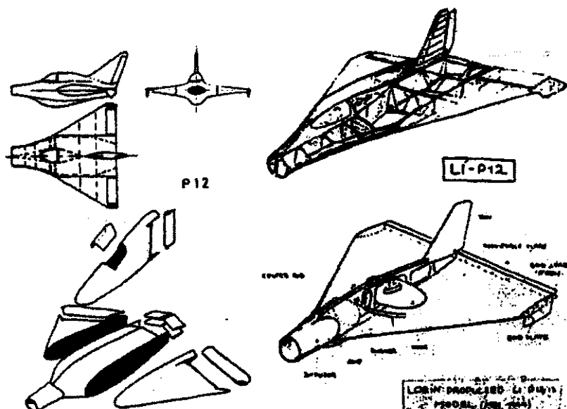
Самолет Липпиша «P-12»
