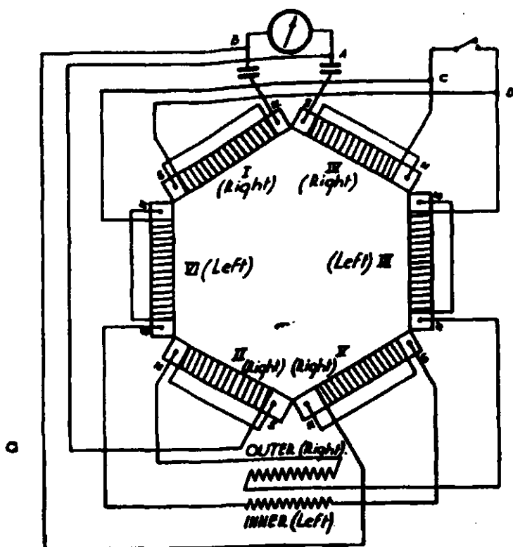
Катушка Колера
