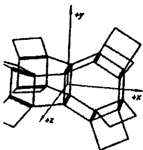
Модель криптона (номер 26, масса 82) Хильгенберга
