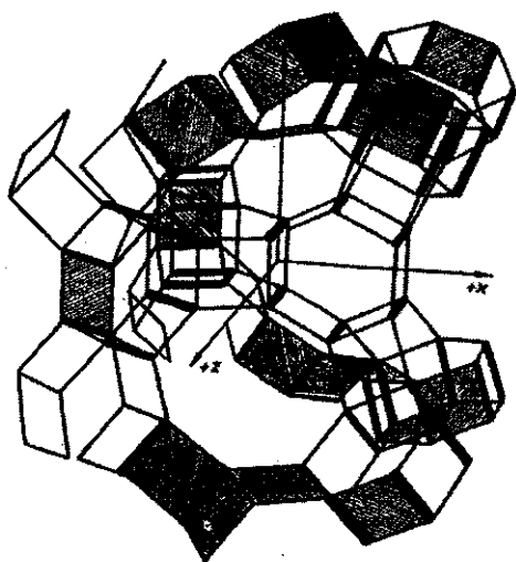
Модель элемента 118, масса 336, Хильгенберга
