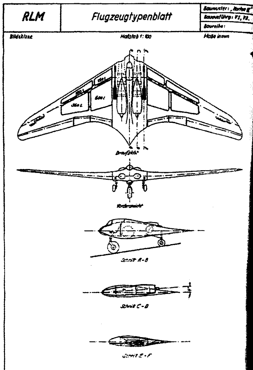
Реактивное «Летучее крыло» братьев Хортен
