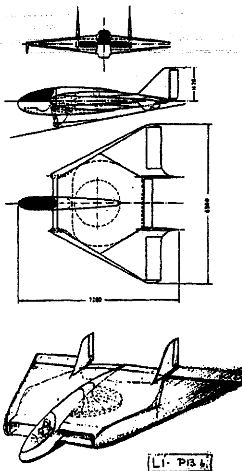
Самолет Липпиша «P-13b»
