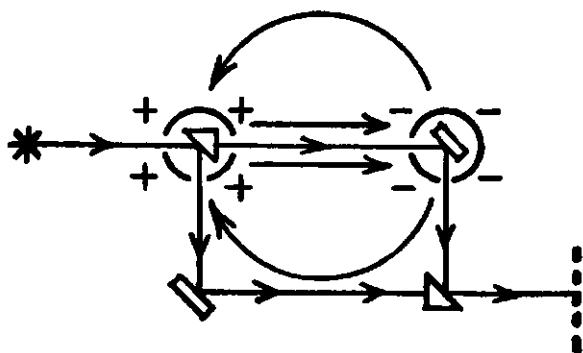
Интерферометр Крафта
