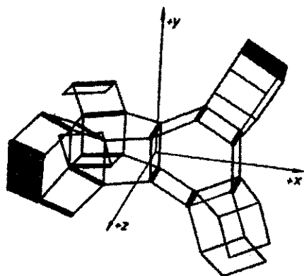
Модель ксенона (номер 54, масса 132) Хильгенберга
