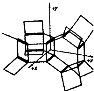
Модель криптона (номер 26, масса 82) Хильгенберга
