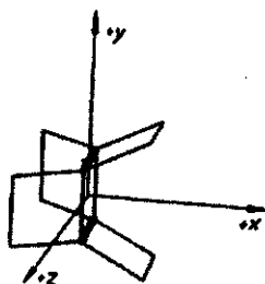
Модель неона (номер 10, масса 22) Хильгенберга
