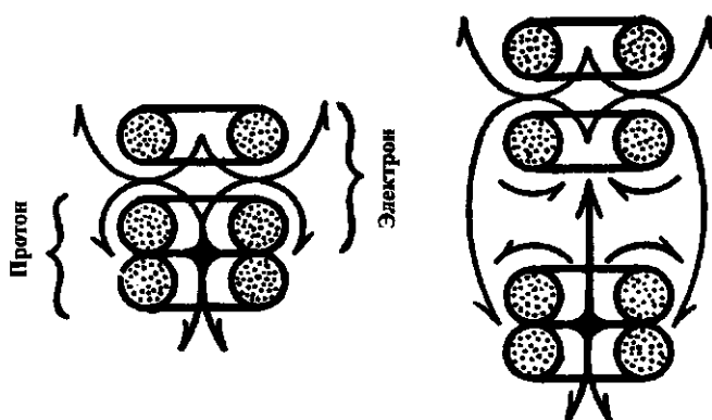
Вихревая модель нейтрона (слева) и атома водорода (справа) Крафта
