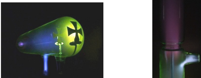
Рисунок 19. «Трубка Крукса» (слева) и каналовые лучи (справа).
