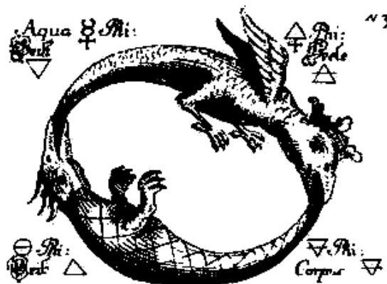
Рисунок 4. Крылатый и бескрылый драконы, образующие круг – алхимические символы Ртути и Серы (Eleazar, Uraltes chymishes Werk , Leipzig, 1760).
