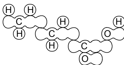
А. Кекуле, 1857-1861
