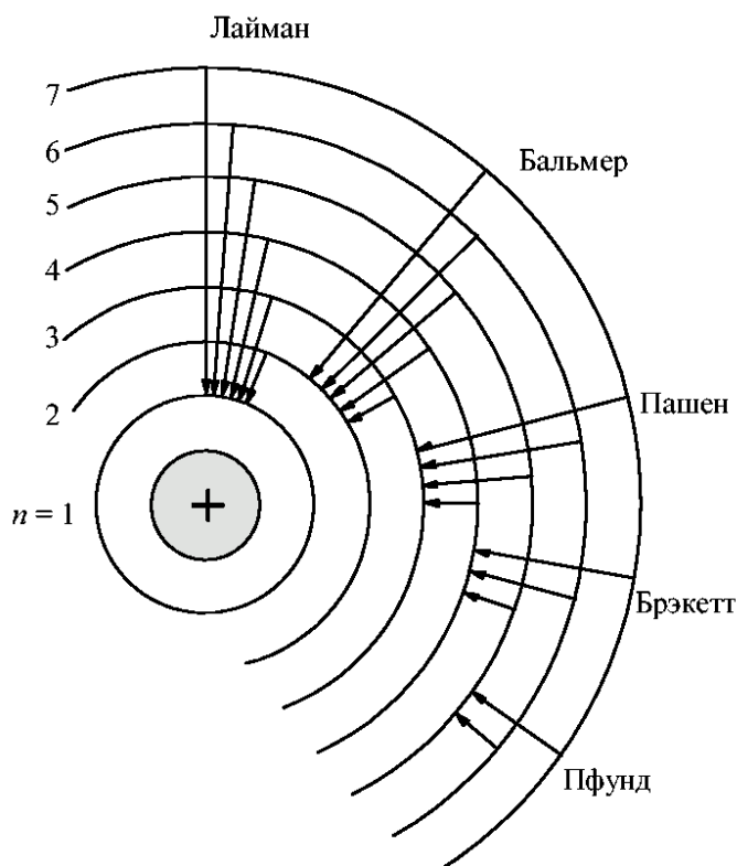
Рисунок 22. Спектральные серии водорода в модели атома Бора.
