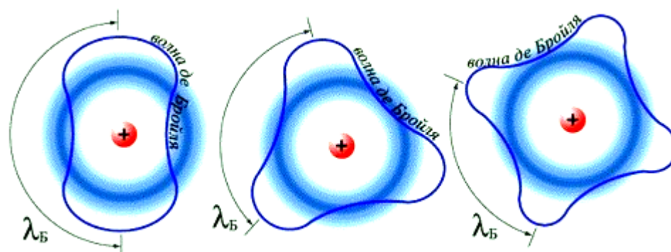
Рисунок 25. Электроны как «волны де Бройля» (главное квантовое число 2, 3 и 4).
