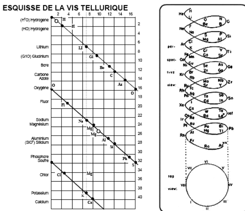
Рисунок 7. «Земная спираль» А. Э. Бегуйе де Шанкуртуа (1862).
