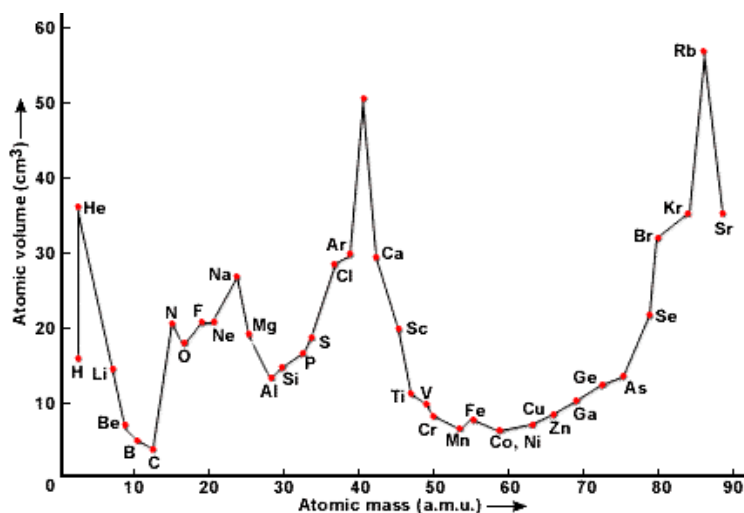
Рисунок 12. Зависимость атомного объема от атомной массы элемента.
