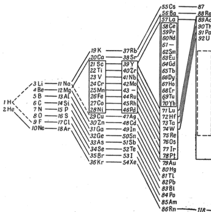
Рисунок 23. «Ступенчатый» вариант периодической таблицы (Н. Бор, 1921).
