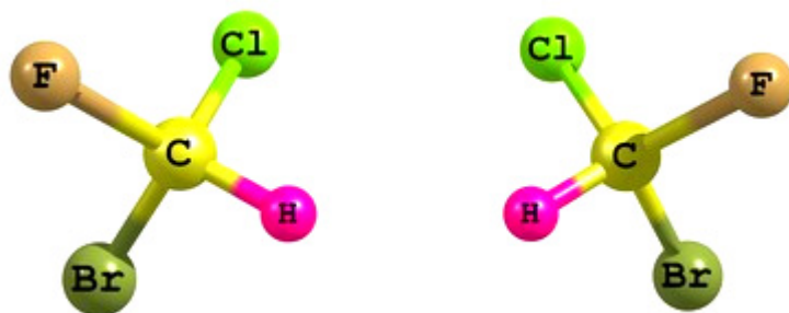
Рисунок 18. Асимметричные (хиральные) атомы углерода.
