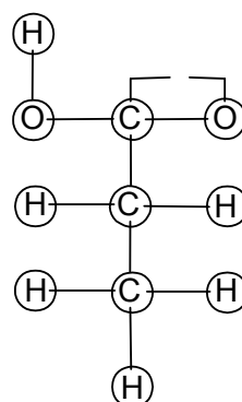
А. Кекуле, 1857-1861
