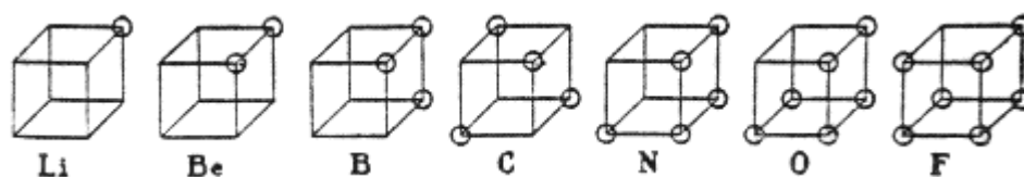
Рисунок 24. «Кубический атом» Льюиса (рисунок из статьи 1916 г.).
