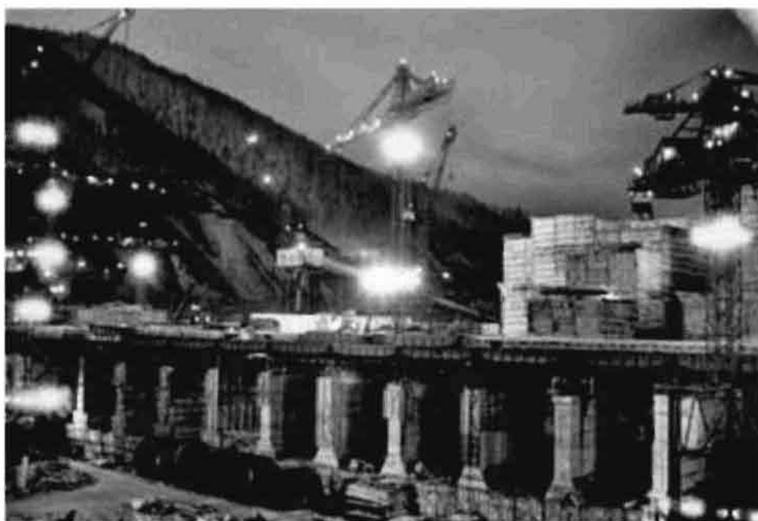
Строительство Красноярской ГЭС — видно, что тело плотины формируется из огромных блоков, каждый из которых заливается по отдельности.
