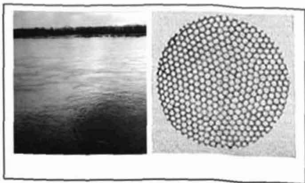
Ячейки на поверхности реки Енисей и вихревые ячейки Бенера (фото автора и иллюстрации из книги: И. Пригожин, «От существующего к возникающему», М., 1983, с. 104).
