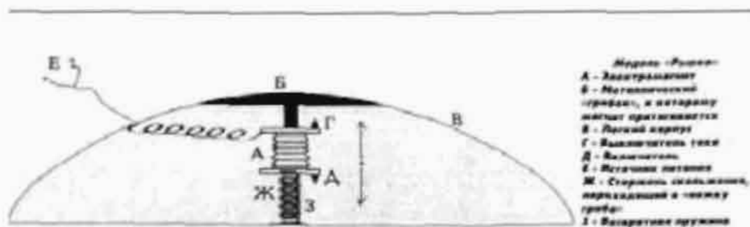
Чертеж модели «рывка» — из статьи «Анатомия летающего обмана». Можете сделать летающую игрушку.
