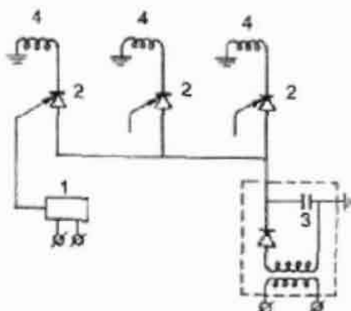
Электрическая схема ЭИПОС. Цифрами обозначены: 1 - программный коммутатор, 2 - тиристор, 3 - конденсатор, 4 - индуктор.
