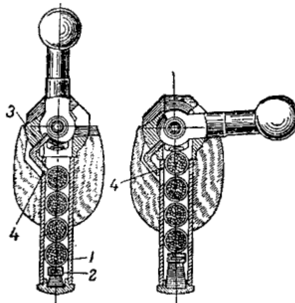
Схема 5. Магазин винтовки образца 1891-1930 гг.: 1 - коробка; 2 - подающий механизм; 3 - отсечка-отражатель; 4 - отсекающий зуб
