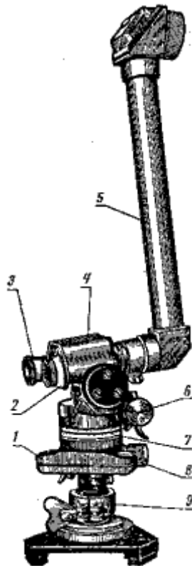
Схема 104. Буссоль 1 - ориентир-буссоль, 2 - привод механизма вертикальной наводки; 3 - окуляр; 4 - оптический визир, 5 - зеркальный перископ, 6 - привод механизма горизонтальной наводки; 7 - шкала; 8 - ориентирующий червяк, 9 - шаровая пята.
