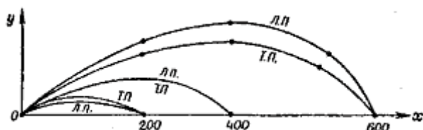
Схема 118. Траектории легкой и тяжелой пули при стрельбе на различные дальности
