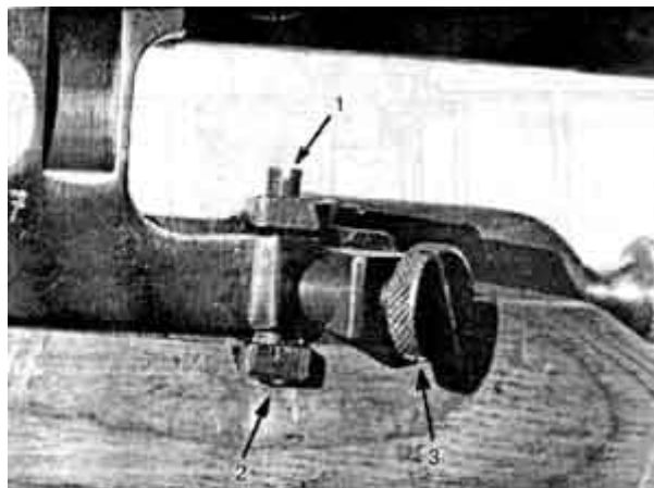
Фото 95. Регулирование системы прицела ПУ: 1 - верхний микрометрический винт;
