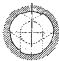
Схема 140. Нарезы 7,5-мм винтовки системы "Шмидт-Рубина" обр. 1889-1896 гг.
