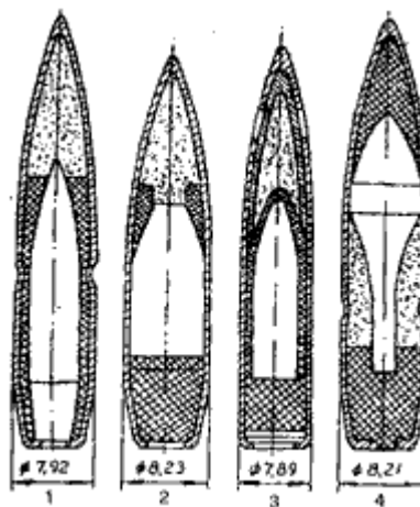
Схема 124 Бронебойно-зажигательные пули:
