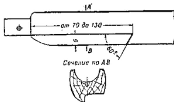
5. Разделка паза для вклейки
