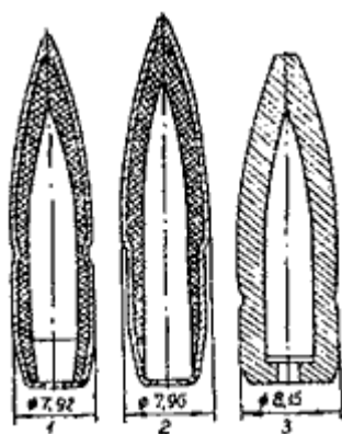
Схема 121. Бронебойные пули:
