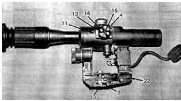
Фото 97. Оптический прицел ПСО-1 (вид справа):
