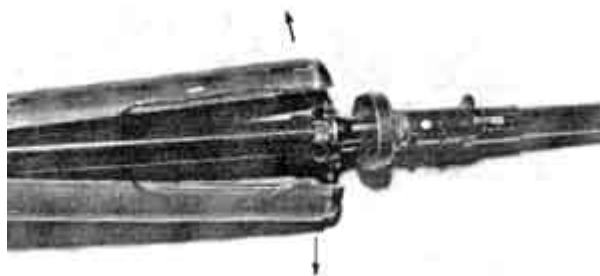
Фото 51. Разборка винтовки: развести в стороны ствольные накладки
