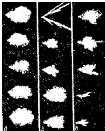
Схема 110. Форс пламени одинаковых капсюлей в разных условиях: А - боек правильной формы и величины при необходимой энергии удара; Б - очень острый и тонкий боек; В - боек нормальной формы при малой энергии удара
