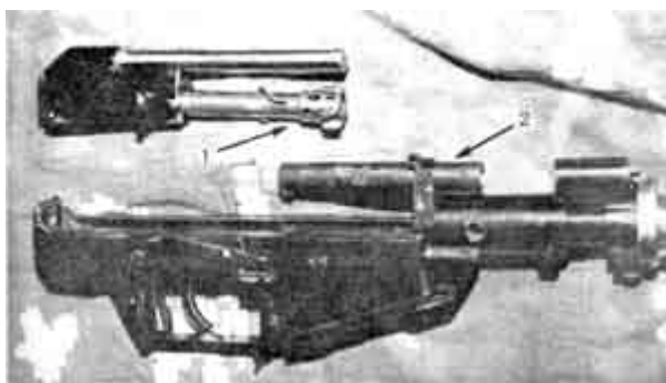
Фото 76. Разборка "Винтореза":
