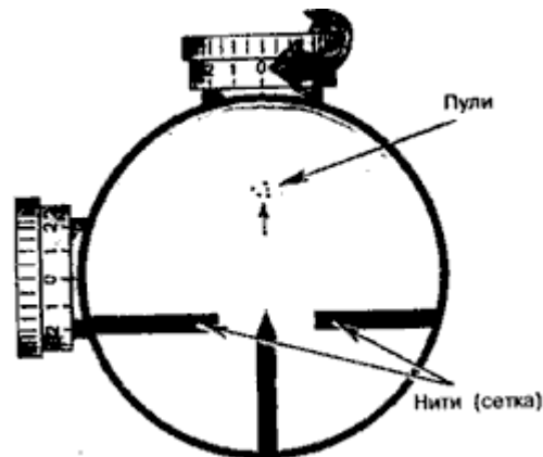
Схема 19. Введение поправок по дальности в прицелах ПУ, ПЕ, ПБ, ПБ. Дистанционный маховик вращается по часовой стрелке, нити (сетка) опускаются вниз, пули уходят вверх
