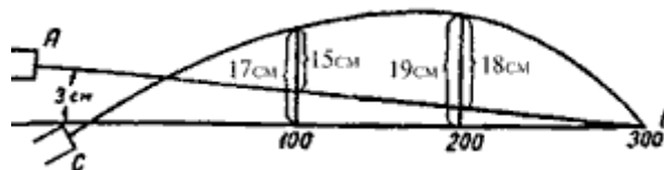
Схема 100. Превышения траектории над линиями прицеливания оптического (AB) и открытого (CB) прицелов
