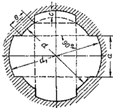
Схема 133. Устройство нарезной части канала ствола (поперечный разрез): а - ширина нарезка; b - ширина поля; c - глубина нарезка; d - калибр оружия; d1 - диаметр по нарезам.
