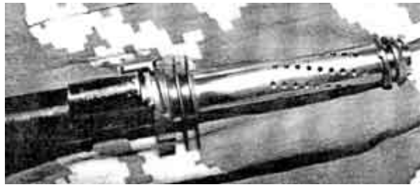
Фото 79. Дырявый ствол бесшумной винтовки
