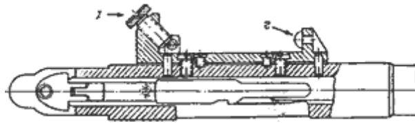
Схема 8. Крепление основания кронштейна прицела ПУ на ствольной коробке 7,62 мм снайперской винтовки 1 - зажимной винт; 2- шаровая опора
