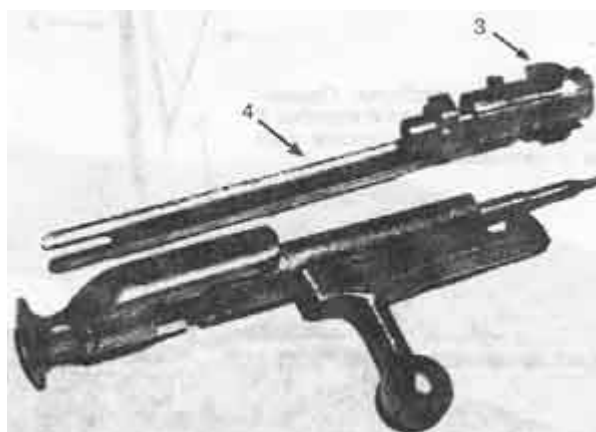
Фото 18. Разборка затвора. Боевую личинку 3 повернуть против часовой стрелки и отделить вперед от соединительной планки 4
