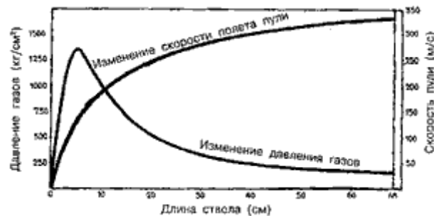
Схема 112. Изменение давления газов и скорости пули в стволе малокалиберной винтовки
