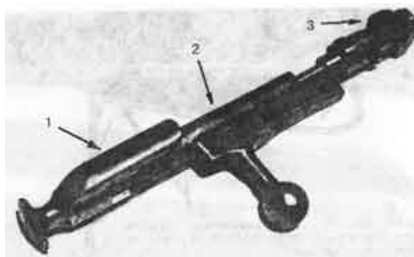
Фото 17. Разборка затвора. Удерживая курок 1, повернуть по часовой стрелке стемпель затвора 2. В таком положении курок спущен. Подать вперед боевую личинку 3
