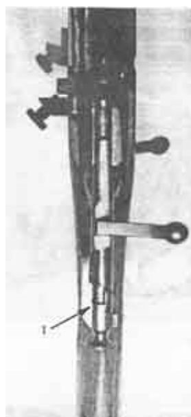
Фото 35. Винтовка, поставленная на длительное хранение. Курок 1 оттянут назад и повернут влево
