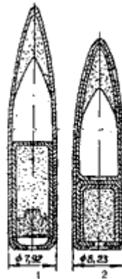
Схема 126. Бронебойно-зажигательно-трассирующие пули:
