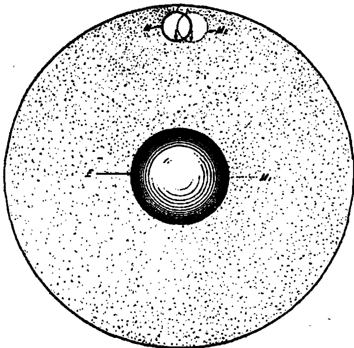
Рис. 12. Концепция Теслы о вращении Луны (М) вокруг Земли (Е). Согласно демонстрируемой здесь гипотезе, Луна рассматривается в качестве тела, погруженного в однородную массу M_1 . Если, как все считают, Луна вращается, это было бы в той же степени верно для части массы M_2 , а часть, общая для обоих тел, вращалась бы одновременно в «противоположных» направлениях.
