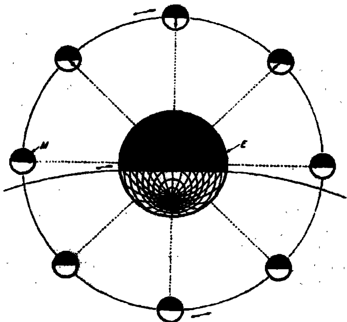
Рис. 11. Хорошо известно, что Луна (М) всегда обращена к Земле (Е) одной и той же стороной, как показывают черные стрелки. Параллельные лучи, исходящие от Солнца, освещают Луну в ее последовательных орбитальных позициях, как показывают незаштрихованные полукруги. Учитывая это, вы действительно полагаете, что Луна вращается вокруг своей оси?
