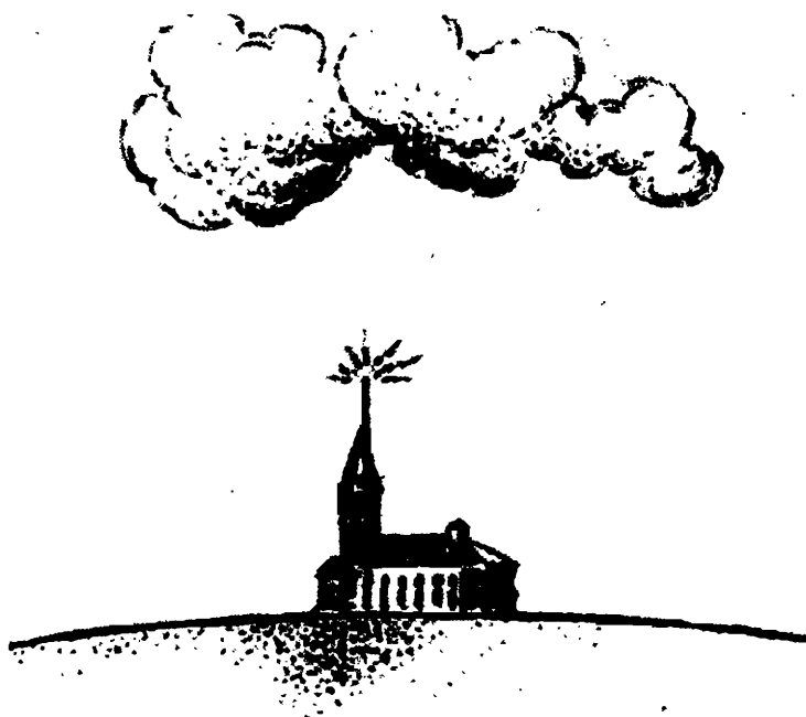
Рис. 14. На этом рисунке Тесла объясняет несостоятельность остроконечного молниеотвода Франклина и показывает, что такой заостренный стержень не смог бы извлечь электричество из одного-единственного облака за долгие годы. Плотность точечной штриховки соответствует силе зарядов.
