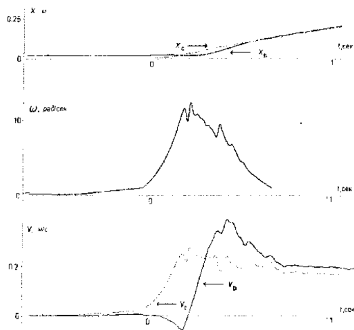
Рис. 26: Экспериментальные графики внутреннего удара 4D гироскопа. v_c - скорость центра масс, v_b - скорость корпуса, \omega - угловая частота вращения грузов
