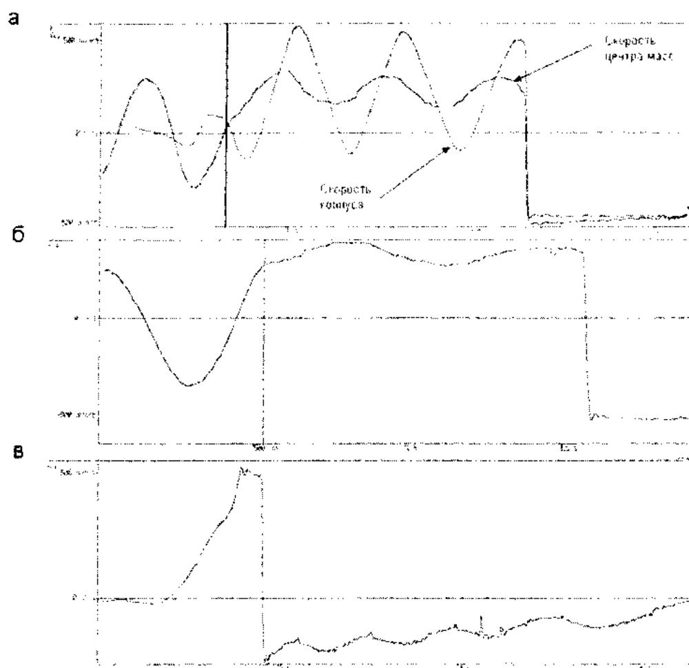
Рис. 19: Экспериментальные наблюдения пространственно-временной прецессии свободного 4D гироскопа в плоскости ct - x во время ударов корпуса о стенку: а) прецессия до удара (после вертикальной линии); б) тоже самое в другом эксперименте; в) прецессия после удара
