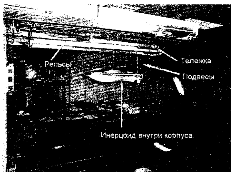
Рис. 7: Эксперимент, предложенный Ж.П.Вижье
