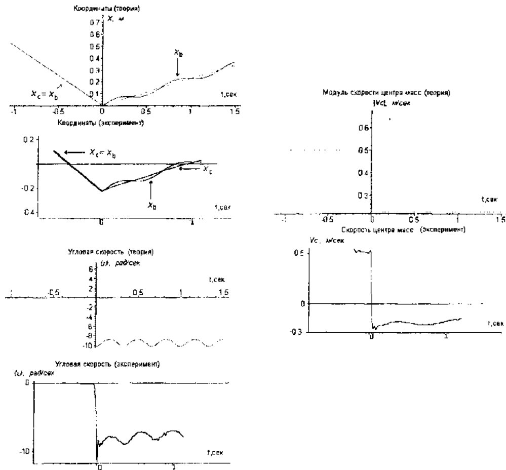
Рис. 22: Сравнение теоретических и экспериментальных данных по короткому упругому удару 4D гироскопа, преобразующему энергию центра масс во вращательную энергию
