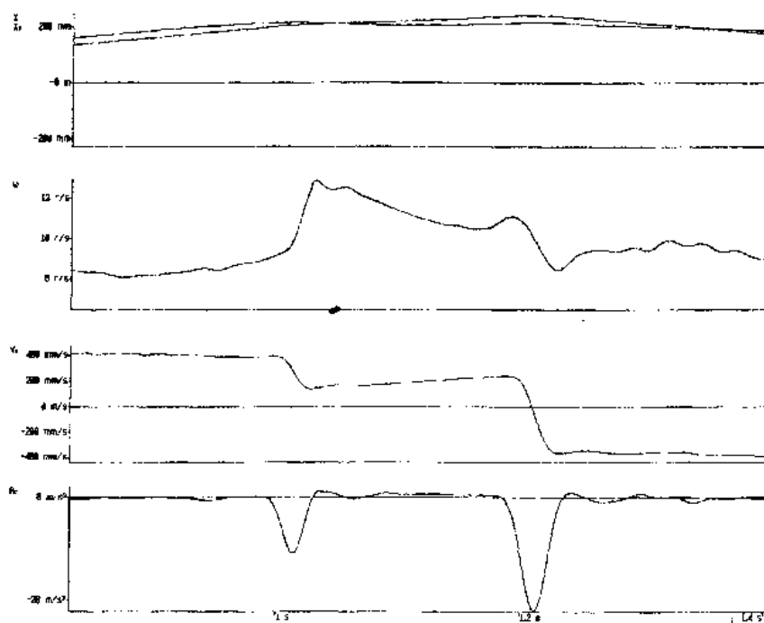
Рис. 25: Двойной удар, демонстрирующий изменение скорости центра масс свободного гироскопа после первого удара
