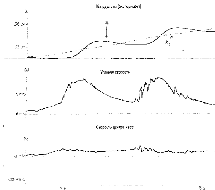
Рис. 28: Экспериментальные графики множественных внутренних ударов 4D гироскопа с пружинным заводом
