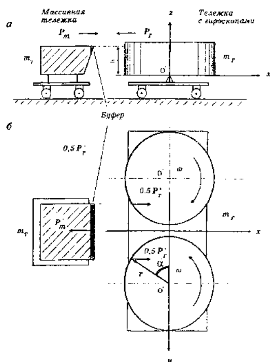
Рис. 32: Столкновение двух гироскопов m_G с массой m_T а – вид сбоку; б – вид сверху
