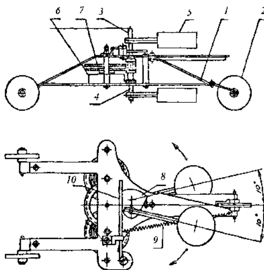
Рис. 2: Схематическое изображение однотактного инерциода
