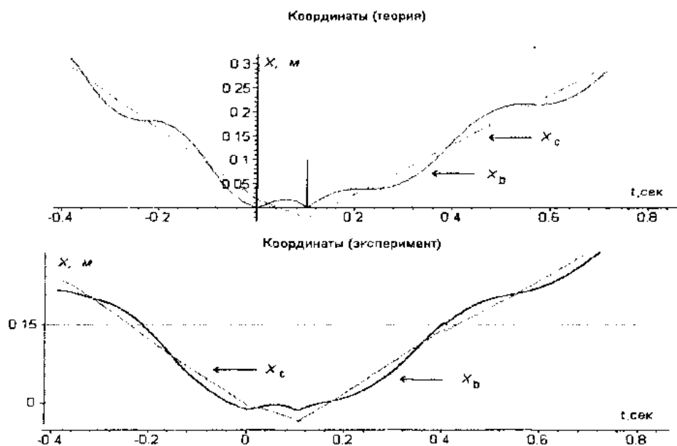
Рис. 24: Теоретический и экспериментальный графики двойного удара
