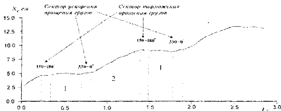
Рис. 4: Движения центра масс инерцоида
