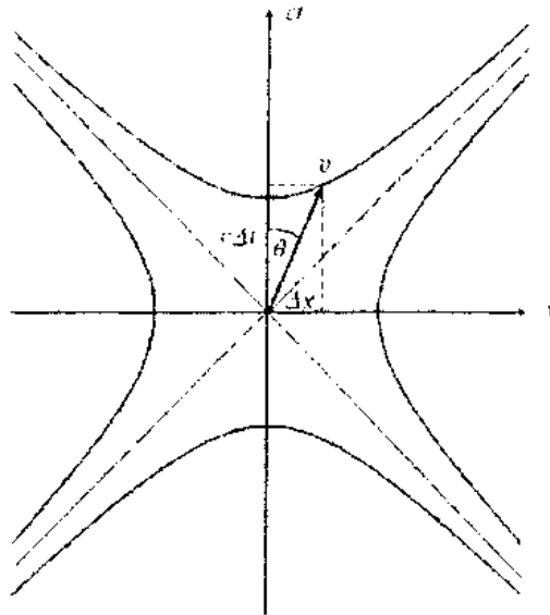
Рис. 15: Поступательное ускорение W_x = dv_x/dt = c(th\theta_x) вдоль оси x есть вращение в плоскости ct - x
