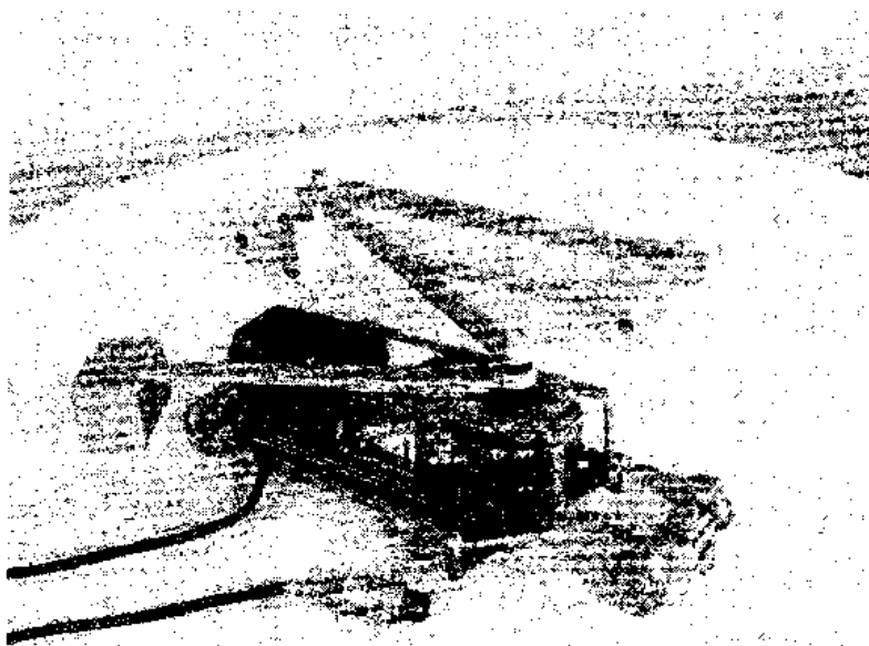
Рис. 9: Мощный инерцоид Толчина с максимальной тягой в импульсе 15 кг.
