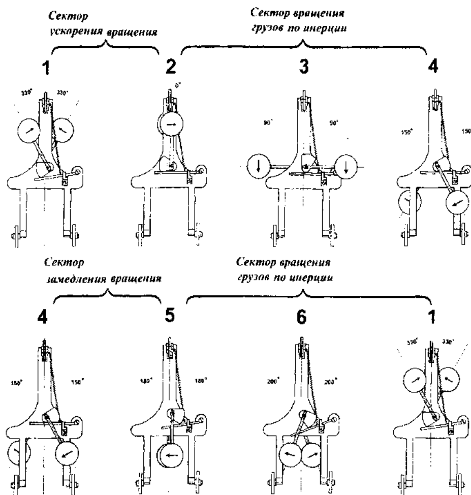
Рис. 3: Действие мотор-тормоза приводит к изменению частоты вращения грузов 5. В секторе углов 330^\circ - 360^\circ угловая скорость увеличивается, а в секторе углов 150^\circ - 180^\circ уменьшается
