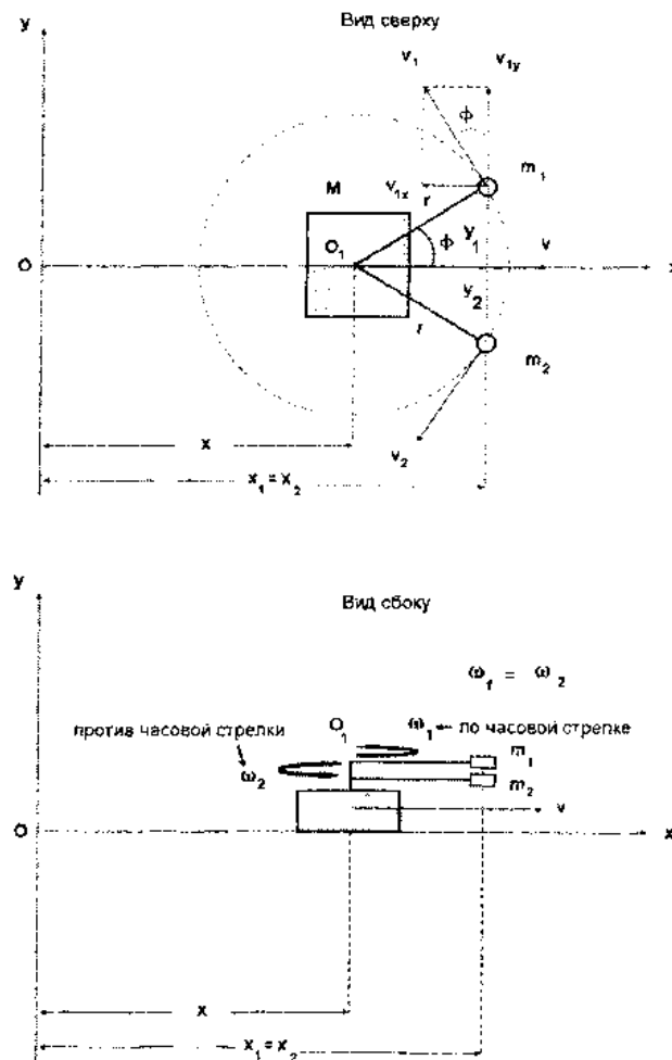
Рис. 12: Принципиальная схема 4-D гироскопа
