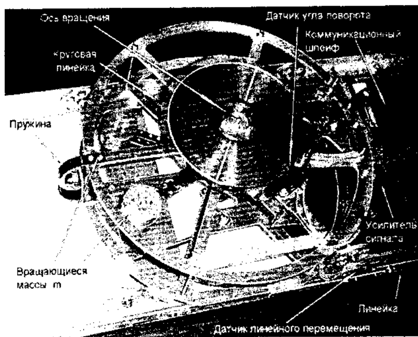
Рис. 20: Четырехмерный гироскоп с системой регистрации движения
