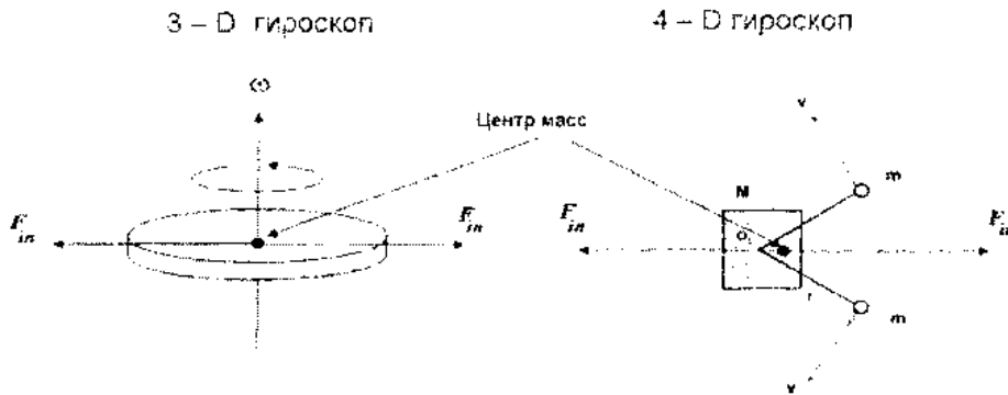
Рис. 17: Примеры локально инерциальной системы отсчета второго рода
