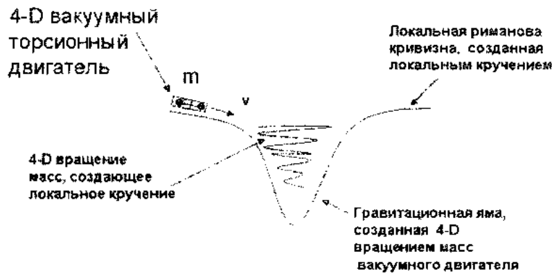
Рис. 33: Движение 4D гироскопа в результате управления локальной метрикой кривизной и кручением пространства событий
