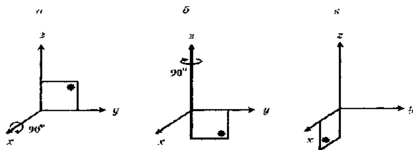
Рис. 14: Смена порядка последовательных поворотов на угол 180^\circ a – поворот по часовой стрелке на угол 90^\circ вокруг оси x ; b – то же, вокруг оси z ; c – результат двух последовательных поворотов
