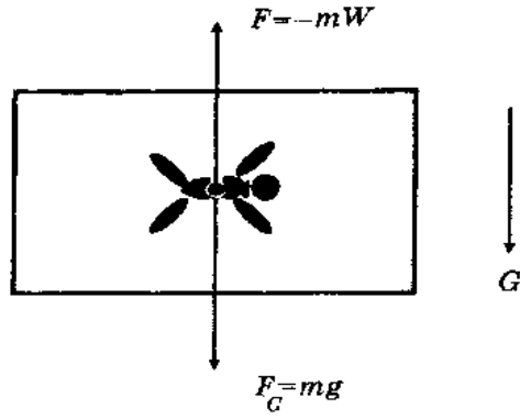
Рис. 16: Пример локально инерциальной системы отсчета первого рода
