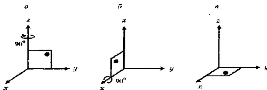
Рис. 13: Два последовательных поворота на угол 180^\circ a – поворот на 90^\circ по часовой стрелке вокруг оси z ; b – то же, вокруг оси x ; c – результат двух последовательных поворотов
