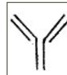
Молекула антитела
