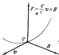
Рис. 2.27. Сила, действующая на положительный заряд q в магнитном поле.
