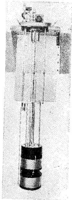
Рис. 1.28. Электромагнит со сверхпроводящими обмотками, работающий при низкой температуре. Эти обмотки рассчитаны на получение магнитного поля в 54 000 гс. Такой прибор является сердцем современной лаборатории низких температур.
