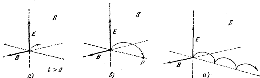
Рис. 4.19. а) Как только заряд q приобретет скорость в направлении E , на него станет действовать сила F=(q/c)\mathbf{v} \times \mathbf{B} . Вследствие этого траектория заряда искривляется в направлении (-y) . б) Заряд q в конце концов попадает в точку P на оси y , где его скорость обращается в нуль. Затем он начинает новый период движения. в) Траектория заряда q представляет собой обычную циклоиду (если в начальном положении он был неподвижен), и заряд q движется со средней скоростью V , направленной вправо: V=cE/B .
