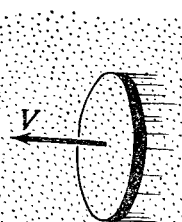
Рис. 7.10. На плоскую пластинку, которая движется в газе, перпендикулярно к ее плоскости при очень низком давлении действует тормозящая сила, пропорциональная ее скорости V (если V значительно меньше, чем средняя скорость молекул газа).
