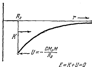
Рис. 5.29. Минимальная кинетическая энергия, необходимая для того, чтобы масса M покинула поверхность Земли (радиуса R_3 ), равна K = \frac{1}{2} Mv_2^2 = \frac{GM_3M}{R_3} ,
