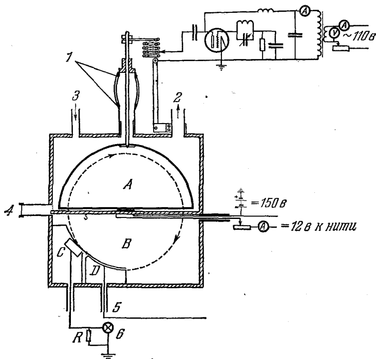
Схема установки для многократного ускорения ионов. 1—соединения медь—стекло 2—вакуумный насос; 3—водород; 4—оконшко; 5—отклоняющий потенциал; 6—электрометр.
