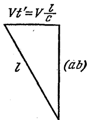
Рис. 10.35. l^2 = \frac{V^2}{c^2} l^2 + (ab)^2 , следовательно, но, l = \frac{(ab)}{(1 - V^2/c^2)^{1/2}} , \Delta t(ab'a') = 2l' = 2(ab)/(c^2 - V^2)^{1/2} .
