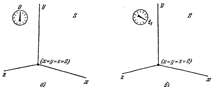
Рис. 11.30. а) Не все интервалы равны нулю. Вот событие: x=y=z=t=0 . б) Вот другое событие: x=y=z=0, t=t_1 . Интервал между этими двумя событиями равен s , где s^2=c^2t_1^2 > 0 . Интервалы, для которых s^2 > 0 , называются времениподобными .
