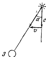
Рис. 10.5. Для наблюдателя, находящегося на Земле (З), свет имеет горизонтальную составляющую скорости v и вертикальную составляющую c . Следовательно, световой луч, идущий от источника, наклонен под углом \alpha , причем \operatorname{tg} \alpha = v/c .
