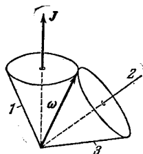
Рис. 8.30. Таким образом, в случае «свободного» вращения аксиально симметричного тела конус тела катится по пространственному конусу (без скольжения). 1 — пространственный конус; 2 — ось симметрии тела; 3 — конус тела.
