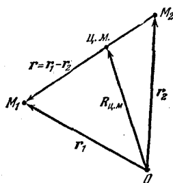
Рис. 9.10. Силы взаимодействия материальных точек M_1 и M_2 — центральные силы, коллинеарные с вектором \hat{\mathbf{r}} ; \mathbf{r}_1 и \mathbf{r}_2 — векторы, описывающие положение M_1 и M_2 в инерциальной системе отсчета с началом в точке O . Если не действуют внешние силы, то \dot{\mathbf{R}}_{\text{ц. м.}} = 0 .
