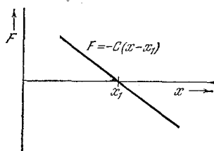
Рис. 5.12. Восстанавливающая сила в пределах малых смещений от x_0 пропорциональна величине смещения.
