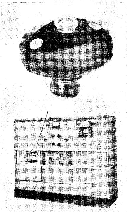
Рис. 3.1. Ротор ультрацентрифуги. Эта ультрацентрифуга работает со скоростью вращения 60 000 об/мин, и в ней возникает центробежное ускорение, превышающее ускорение силы тяжести почти в 300 000 раз.
