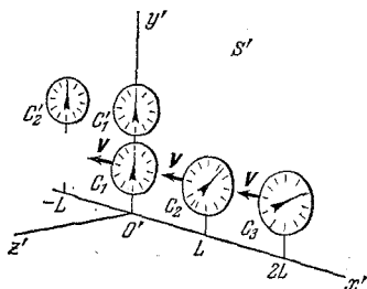
Рис. 11.16. В системе отсчета S' часы C_1, C_2 и т. д. неподвижны, расположены друг от друга на расстояниях L и синхронизированы. Для наблюдателя в системе S часы C_1, C_2, C_3 не синхронизированы! Что они показывают?
