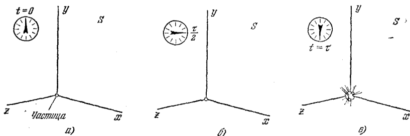
Рис. 11.18. Другой пример замедления времени: а) нестабильная частица неподвижна в системе отсчета S . Мы начинаем наблюдать за ней в момент t=0 . Проходит время (б), и частица распадается (в) в момент t=\tau .
