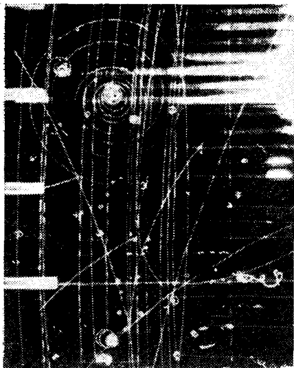
Рис. 15.14. Мезоны с «друзьями» в водородной пузырьковой камере. (Радиационная лаборатория им. Лоуренса)
