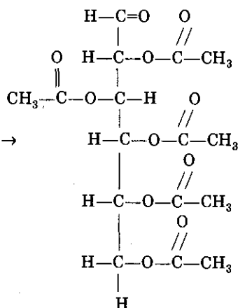
пентаацетилглюкоза
