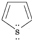
тиофен
