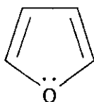
фуран
