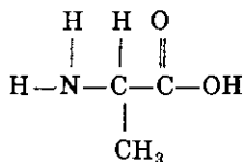
аланин
