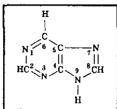
пури́н
