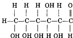
аланин
