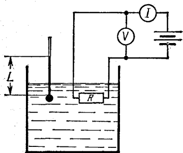
Рис. 1.32. Два различных термометра находятся в тепловом контакте с системой, состоящей из сосуда, наполненного жидкостью. Один термометр ртутный и его термическим параметром является длина столбика ртути в стеклянном капилляре термометра. Другой термометр представляет собой электрическое сопротивление R , сделанное из платиновой проволоки или из угля. Его термическим параметром является электрическое сопротивление R (определяемое током I , текущим через сопротивление, и напряжением V на нем).
