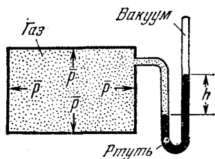
Рис. 1.33. Среднее давление газа \bar{p} измеряется при помощи манометра, состоящего из U-образной трубки, наполненной ртутью. В трубке устанавливается такая высота h столбика ртути, чтобы давление, оказываемое этим столбиком, уравновешивалось давлением газа.
