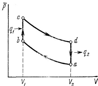
Рис. 7.17. Упрощенная схема работы бензинового двигателя в переменных: среднее давление \bar{p} , объем V .
