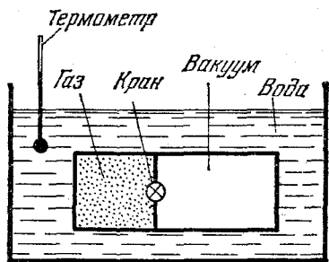
Рис. 5.19. Прибор для изучения свободного расширения газа.
