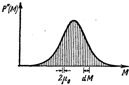
Рис. 2.11. Вероятность P''(M) того, что полный магнитный момент системы спинов имеет значение M , для случая, когда число N спинов велико и магнитный момент спина \mu_0 относительно мал.
