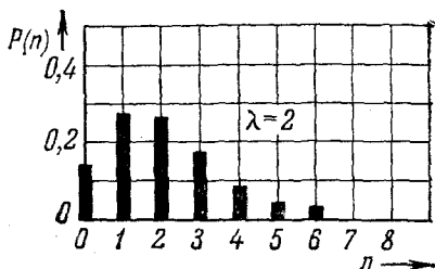
Рис. П.2. Распределение Пуассона P(n) как функция n . Два случая соответствуют средним значениям \bar{n} = \lambda = 1/2 и 2.
