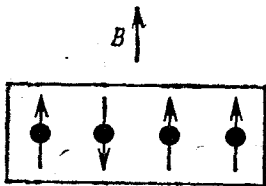
Рис. 2.5. Система из N спинов, равных 1/2 , в частном случае N=4 . Каждая стрелка показывает направление магнитного момента спина. Внешнее магнитное поле обозначено стрелкой \mathbf{B} .
