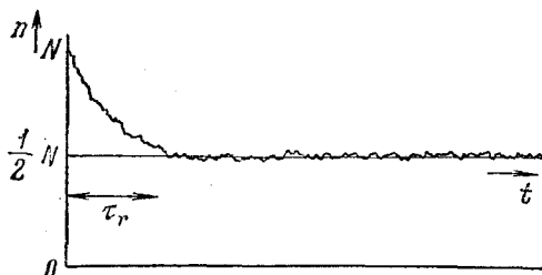
Рис. 1.12. Диаграмма показывает изменение со временем числа молекул n в левой половине ящика на рис. 1.11 после поднятия перегородки. Время релаксации обозначено через \tau_r .
