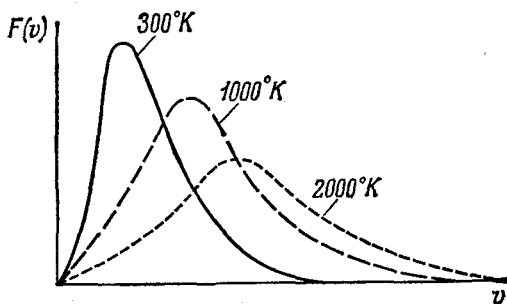
Рис. 6.8. Максвелловское распределение скоростей молекул при различных температурах.
