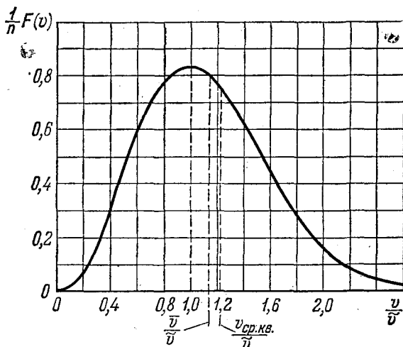
Рис. 6.7. Максвелловское распределение, показывающее среднее число молекул F(v)dv в единице объема, имеющих скорость от v до v+dv . За единицу скорости взята наиболее вероятная скорость \bar{v}=(2kT/m)^{1/2} . На графике показана средняя скорость \bar{v} и средняя квадратичная скорость v_{\text{ср.кв.}}=(v^2)^{1/2} .
