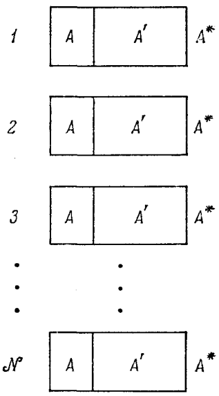
Рис. 3.11. Ассамблея систем A^* : Каждая система A^* состоит из двух систем, A и A' , которые могут взаимодействовать друг с другом.
