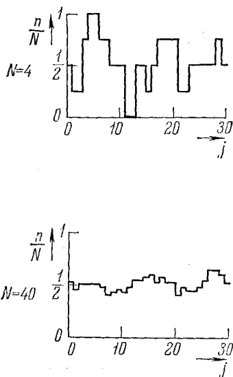
Рис. 1.6. Относительное число n/N частиц в левой половине ящика в зависимости от номера кадра j или текущего времени t=j\tau_0 . Эти графики содержат ту же информацию, что и рис. 1.5
