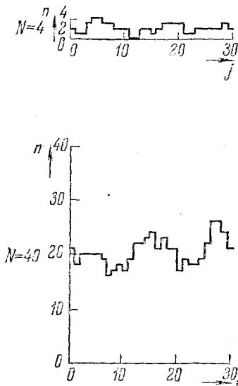
Рис. 1.5. Число n частиц в левой половине ящика в зависимости от номера кадра j или текущего времени t=j\tau_0 . Число частиц на кадре представлено горизонтальной чертой, простирающейся от j до j+1 . Графики иллюстрируют рис. 1.3 для N=4 и рис. 1.4 для N=40 , но содержат информацию о большем числе кадров, чем показано на этих рисунках.
