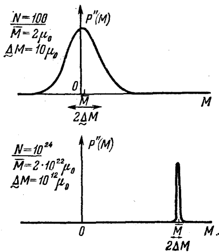
Рис. 2.9. Вероятность P''(M) того, что полный магнитный момент системы спинов имеет значение M , для N=100 и N=10^{24} . Магнитное поле таково, что p=0,51 и q=0,49 . Графики являются огибающими кривыми возможных значений P''(M) . Графики имеют разные масштабы.
