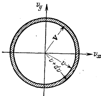
Рис. 6.6. Пространство скоростей для двух измерений (ось v_y перпендикулярна к плоскости чертежа). Сферический слой содержит все молекулы, скорость которых v такова, что v < |\mathbf{v}| < v + dv .
