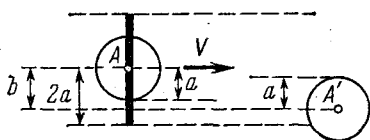
Рис. 1.35. Рисунок иллюстрирует столкновение двух тяжелых сфер радиусом a .
