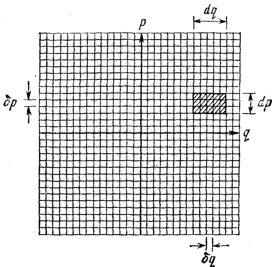
Рис. 6.4. Пример двумерного фазового пространства, разделенного на малые ячейки равного «объема» \delta q \delta p = h_0 . Заштрихованная область соответствует элементу объема величиной dq dp , содержащему много ячеек.
