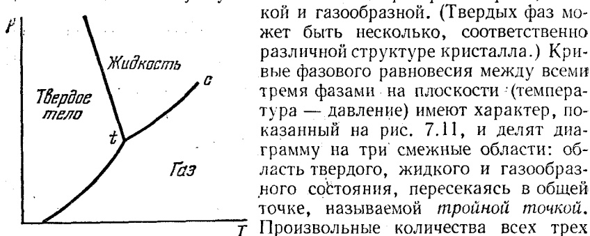
Рис. 7. 11. Фазовая диаграмма вещества, подобного воде. Через t обозначена тройная точка, c — критическая точка.
