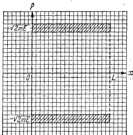
Рис. 6.3. Классическое фазовое пространство частицы, движущейся в одном измерении в ящике длиной L . Состояние частицы характеризуется координатой x и импульсом p ; ее энергия лежит между E и E+dE . Состояния, доступные частице, соответствуют ячейкам, находящимся в заштрихованных областях.
