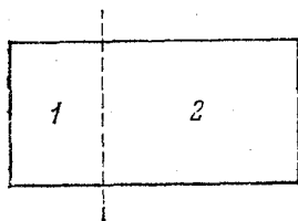
Рис. 5.15. Разделение однородной макроскопической системы на две части
