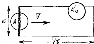
Рис. 8.2. Схема, иллюстрирующая столкновение молекулы A с другой молекулой, центр которой попадает в объем, образованный движением поверхности \sigma воображаемого диска, несомого молекулой A .
