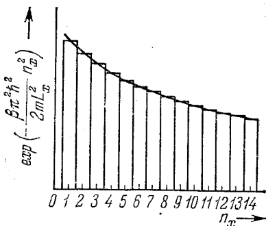
Рис. 4.11. Схема, иллюстрирующая замену суммирования по целым значениям n_x (сумма равна площади прямоугольников) интегрированием по непрерывным значениям переменной n_x (интеграл равен площади под кривой).
