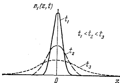
Рис. 8.10. Число n_1(z, t) меченых молекул в единице объема как функция координаты z в различные моменты времени. При t=0 молекулы расположены вблизи плоскости z=0 . Поверхность под всеми кривыми одна и та же и равна полному числу N_1 меченых молекул.
