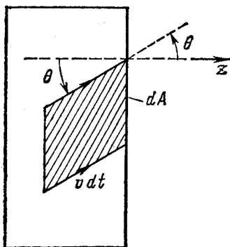
Рис. П.3. Столкновение молекул, скорости которых лежат между v и v+dv , с элементом поверхности dA стенки. (Заметьте, что высота цилиндра стремится к нулю, если dt \rightarrow 0 .)
