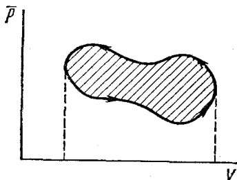
Рис. 5.17. Циклический процесс.
