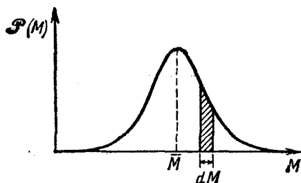
Рис. 2.12. Распределение вероятности, показанное на рис. 2.11, выражено через плотность вероятности \mathcal{P}(M) . Теперь \mathcal{P}(M)dM (площадь под кривой, заключенная между координатами M и M + dM ) есть вероятность того, что полный магнитный момент лежит в интервале значений от M до M + dM
