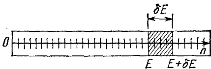
Рис. 3.6. Метки на прямой обозначают возможные значения n=1, 2, 3, 4, \dots квантового числа n , определяющего состояние одиночной частицы в одномерном ящике. Значения n , соответствующие энергиям E и E+\delta E обозначены двумя вертикальными линиями, и область между этими линиями включает в себе все значения n , для которых энергия лежит в интервале от E до E+\delta E . Область слева от E включает в себе все значения n , для которых энергия частицы меньше E .
