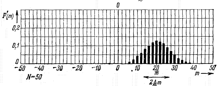
Рис. 2.8. Вероятность P'(m) того, что полный магнитный момент системы из N спинов 1/2 равен m (если его измерять в единицах \mu_0 ). Из-за наличия магнитного поля p=0.7 и q=0.3 . Графики дают значение P'(m) для четырех различных случаев, соответствующих N=10, 20, 30 и 50 .
