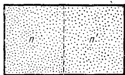
Рис. 1.1. Ящик, в котором находится идеальный газ из N молекул. Ящик разделен на две части воображаемой плоскостью. Число молекул в левой половине n , число молекул в правой половине n' .
