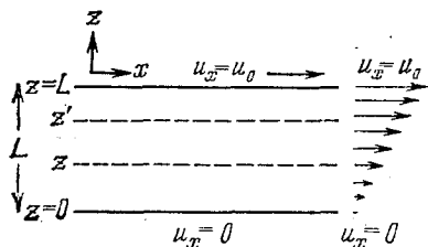
Рис. 8.4. Жидкость, заключенная между двумя пластинами. Нижняя пластина неподвижна, а верхняя движется со скоростью u_0 в направлении x ; таким образом, в жидкости существует градиент скорости \partial u_x / \partial z .
