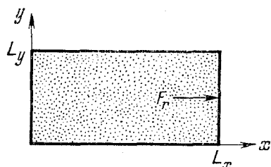
Рис. 4.12. Идеальный газ в ящике. Молекула, находящаяся в состоянии r , действует на правую стенку ящика с силой, проекция которой на ось x равна F_r .
