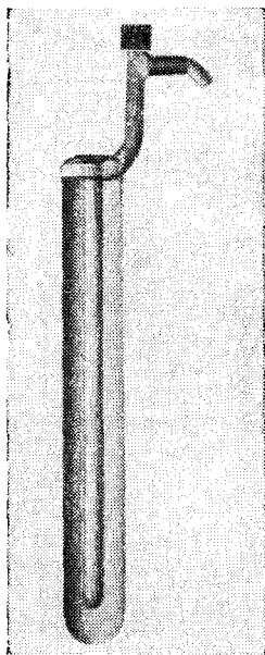
Рис. 5.2 Фотография типичной ячейки для получения тройной точки воды, используемой в Национальном Бюро стандартов.
