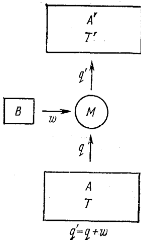
Рис. 7.15. Схема работы холодильника.
