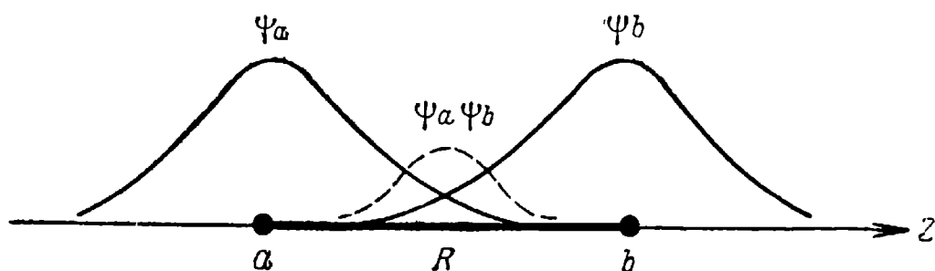
Рис. 16. Наложение атомных волновых функций в молекуле водорода.
