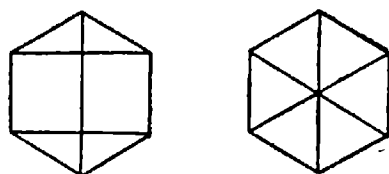
Рис. 39. Структурные формы с перекрещиванием связей.
