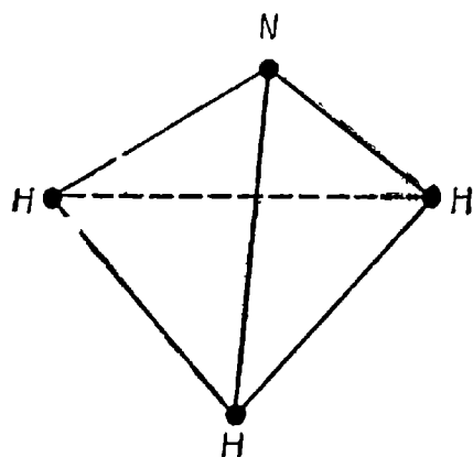
Рис. 22. Расположение атомов в молекуле аммиака.
