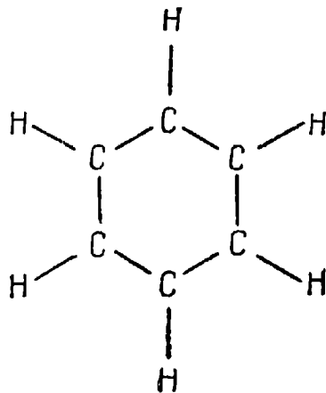
Рис. 36. Расположение атомов и \sigma -связей в молекуле бензола.
