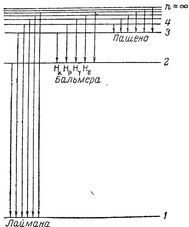
Рис. 4. Схема энергетических уровней атома водорода и происхождение спектральных серий.
