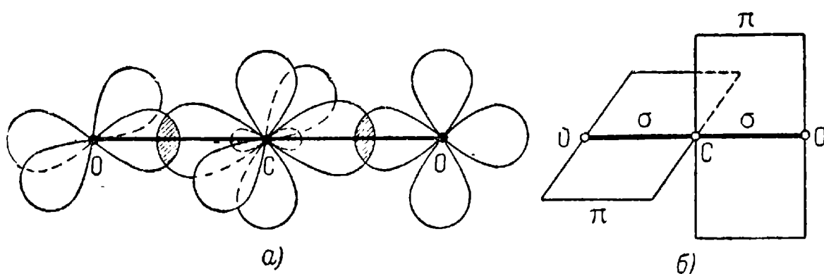
Рис. 34. Молекула углекислого газа: a — расположение облаков валентных электронов, б — схема валентных связей.
