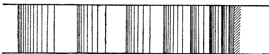
Рис. 48. Электронно-колебательный спектр поглощения.
