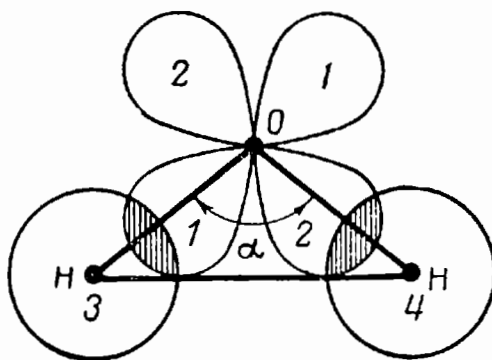
Рис. 21. Форма и расположение одноэлектронных атомных облаков в молекуле воды.
