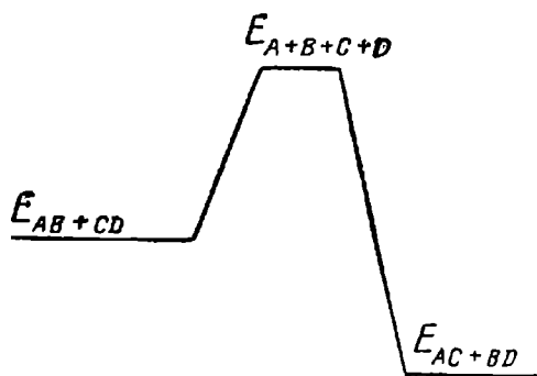
Рис. 53. Схема потенциального барьера в реакции обмена.
