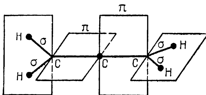
Рис. 35. Схема валентных связей в молекуле аллена.
