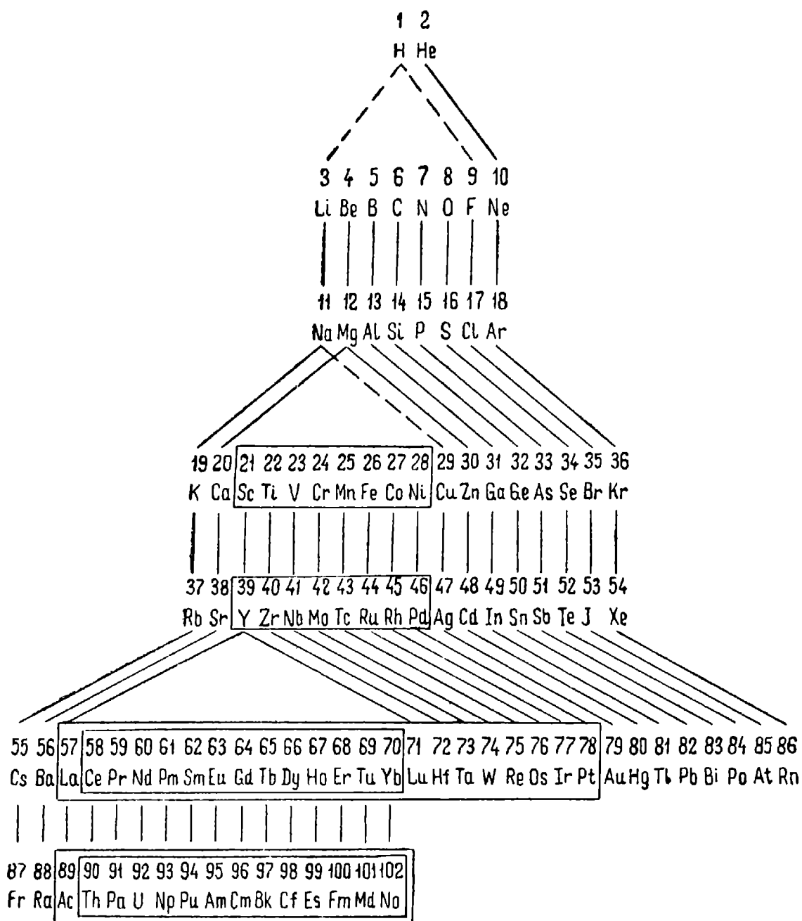
Рис. 13. Периодическая система элементов.
