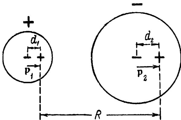
Рис. 45. Индуцирование атомных диполей при взаимодействии ионов.
