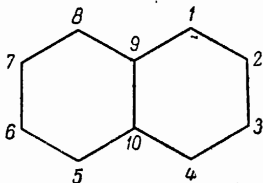
Рис. 55. Нумерация атомов в молекуле нафталина.
