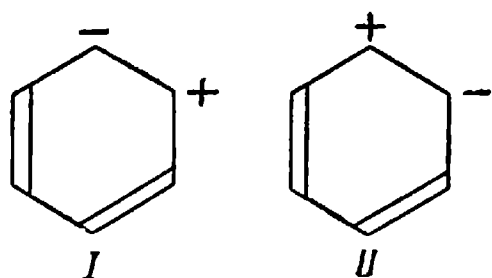
Рис. 43. Ионные валентные схемы бензола.
