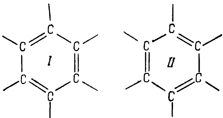
Рис. 37. Структурные формы Кекуле.
