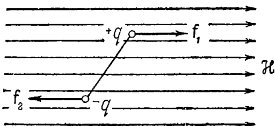
Рис. 5. Магнитный диполь в однородном магнитном поле.
