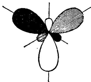
Рис. 30. Форма и расположение облаков вероятности электронов в случае sp^2 -гибридизации.
