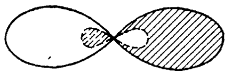
Рис. 32. Форма и расположение электронного облака при sp -гибридизации.
