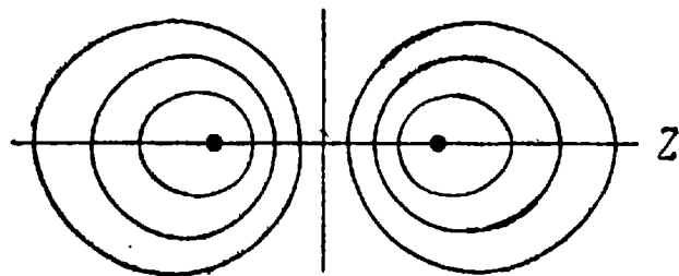
Рис. 18. Линии постоянной плотности вероятности р-электрона.
