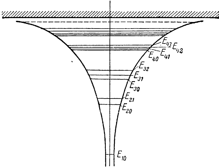
Рис. 11. Относительное расположение уровней энергии электрона в центральном поле атома.
