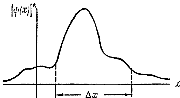
Рис. 9. Распределение вероятностей координат частицы в некотором состоянии.
