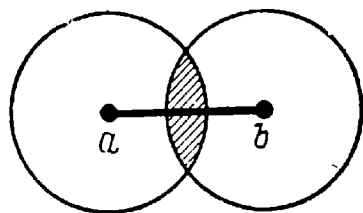
Рис. 17. Форма перекрывания электронных облаков s -состояний.
