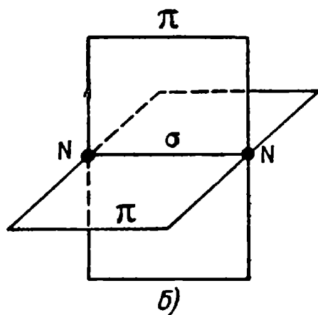
Рис. 26. Молекула азота: а — расположение облаков валентных электронов, б — схема валентных связей.
