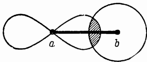
Рис. 20. Форма перекрывания электронных облаков s- и p-состояний.
