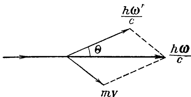
Рис. 1. Сохранение количества движения в явлении Комптона.
