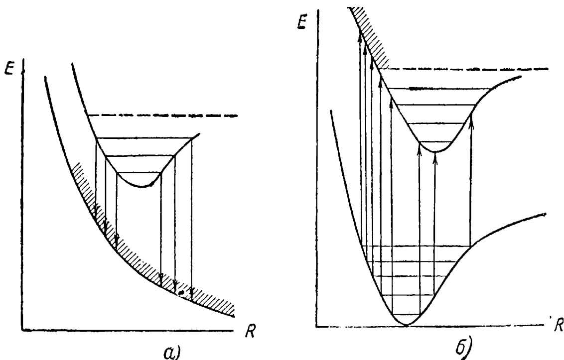
Рис. 50. Электронные переходы в молекуле, дающие сплошной спектр: a — переход из устойчивого состояния в отталкивательное, б — переход между двумя состояниями, обладающими минимумом потенциальной кривой.
