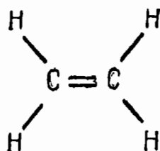
Рис. 29. Структурная формула этилена.
