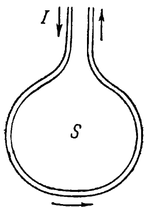
Рис. 6. Проволочный контур с током.
