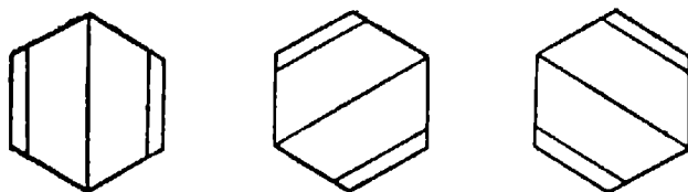
Рис. 38. Структурные формы Дьюара.
