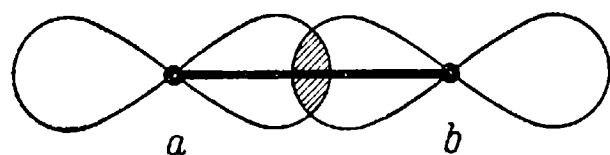
Рис. 23. Расположение одноэлектронных облаков р-электронов, образующих \sigma -связь.
