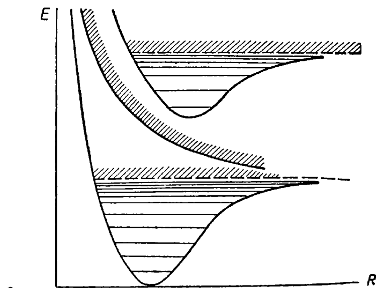
Рис. 47. Потенциальные кривые двухатомной молекулы.
