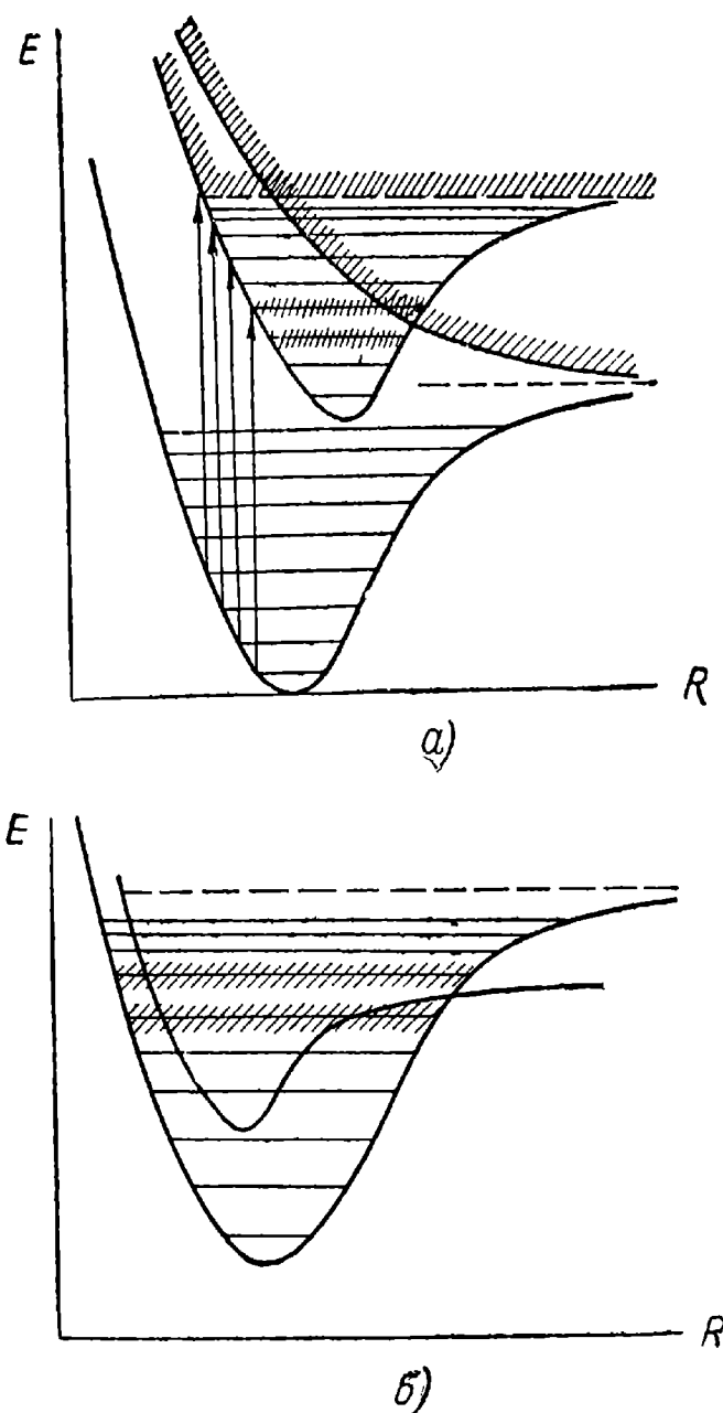
Рис. 51. Различные типы пересечения потенциальных кривых.
