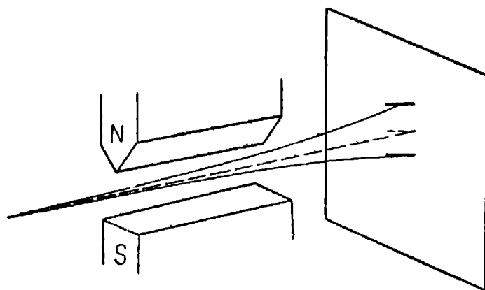
Рис. 7. Расщепление атомного пучка в неоднородном магнитном поле.
