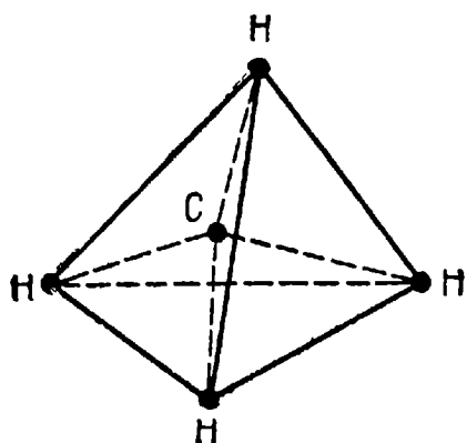
Рис. 27. Расположение атомов в молекуле метана.
