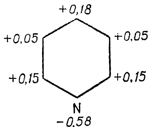
Рис. 56. Полные заряды на атомах молекулы пиридина.
