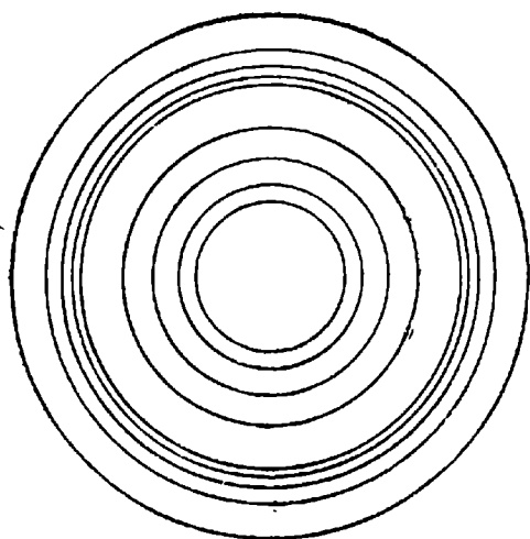
Рис. 8. Дифракционные кольца при прохождении электронов сквозь металлическую пластинку.
