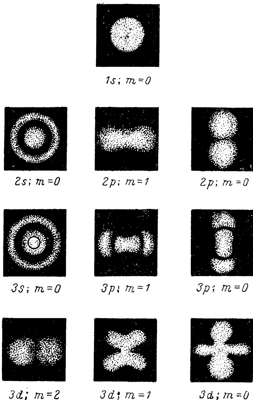
Рис. 12. Электронное облако вероятности первых s-, p-, d-состояний.
