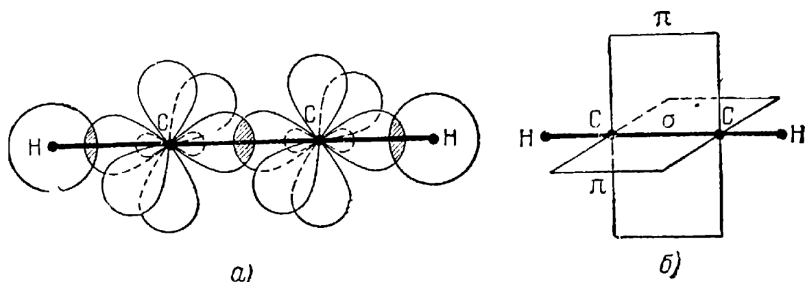
Рис. 33. Молекула ацетилена: a — расположение облаков валентных электронов, б — схема валентных связей.
