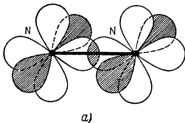
Рис. 26. Молекула азота: а — расположение облаков валентных электронов, б — схема валентных связей.
