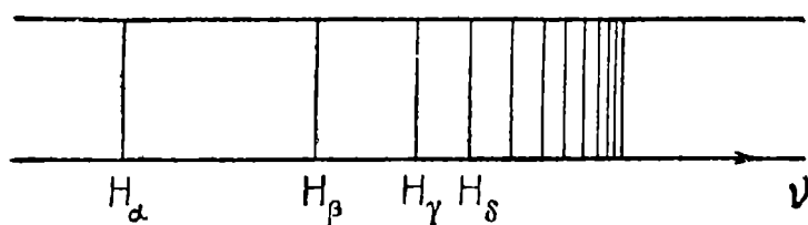
Рис. 2. Расположение спектральных линий серии Бальмера.
