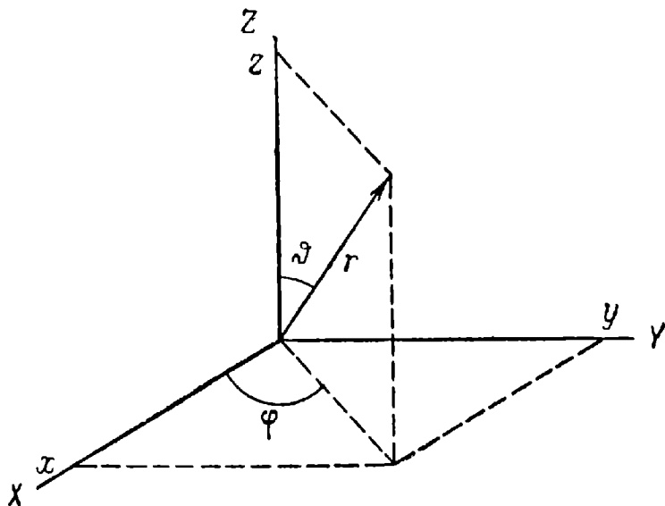
Рис. 10. Прямоугольные и сферические координаты.
