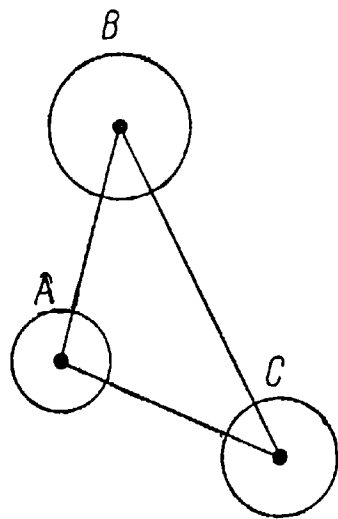
Рис. 54. Конфигурация трех атомов в реакции замещения.
