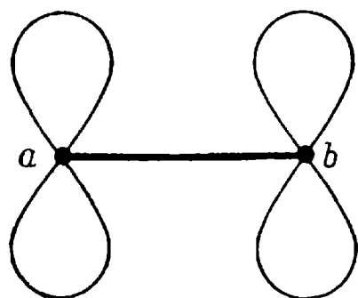
Рис. 25. Расположение облаков вероятности электронов, образующих \pi -связь.
