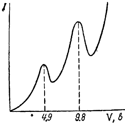
Рис. 3. Результаты опытов Франка и Герца с пропусканием электронов сквозь пары ртути.
